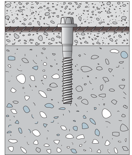
Connettore a vite con parte filettata lunga 65 mm.
