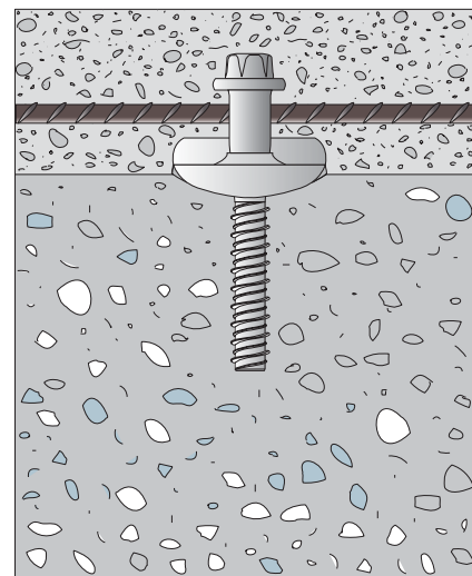
Connettore fornito completo piastra dentata e di vite con parte filettata lunga 65 mm.
