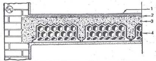
Fig. 42 - PLANCHER EN BÉTON ARMÉ ET BRIQUES CREUSES COMMUNES - 1 Sol - 2 Sous-couche - 3 Coulage du béton - 4 Briques creuses.
