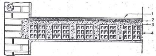
Fig. 42 - PLANCHER EN BÉTON ARMÉ ET BRIQUES CREUSES COMMUNES - 1 Sol - 2 Sous-couche - 3 Coulage du béton - 4 Briques creuses.
